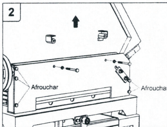
Afrouxe os parafusos indicados, desparafuse e retire as 4 guias.
